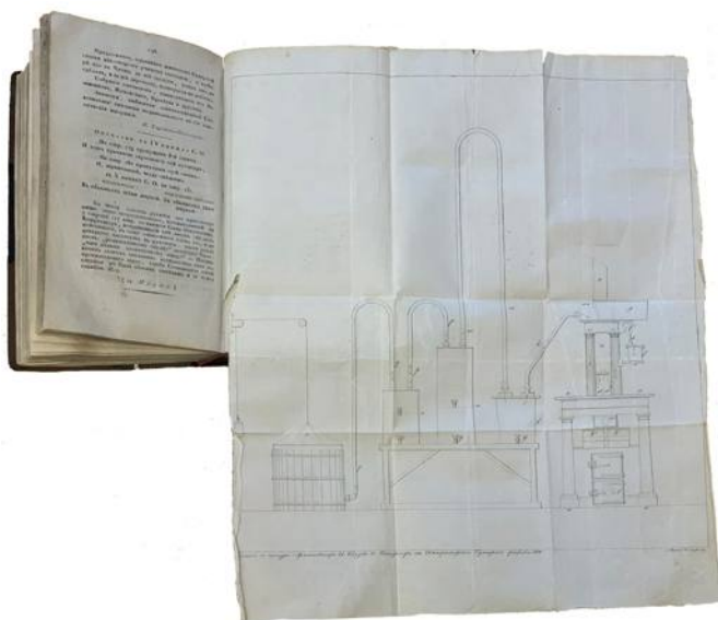
Рис. 10. Рис. И. Связов, лит. К.П. Бегров. Рисунок с препаратов, устроенных на Императорской бумажной фабрике в Петергофе, для делания масляного газа («Сын Отечества», 1821 г., Ч. 68, № 11). Литография. Лист – 31,5 х 37,7 см. Фото автора статьи
